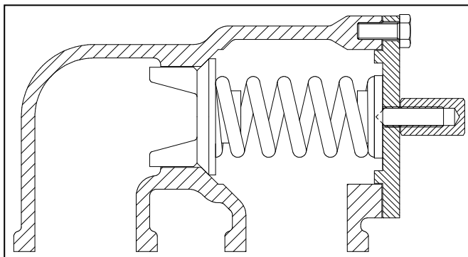
Figura 3 - Valvola di sicurezza (by-pass)
