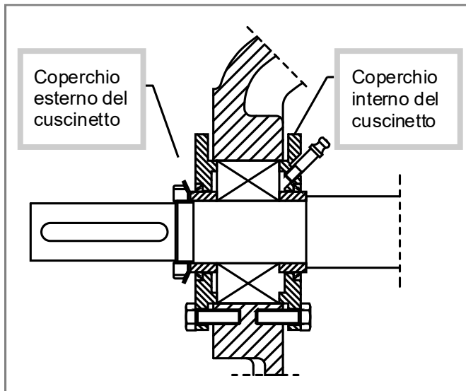
Figura 2 - Coperchi del cuscinetto
